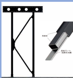
▲先進技術を採用した高耐力制震フレーム
